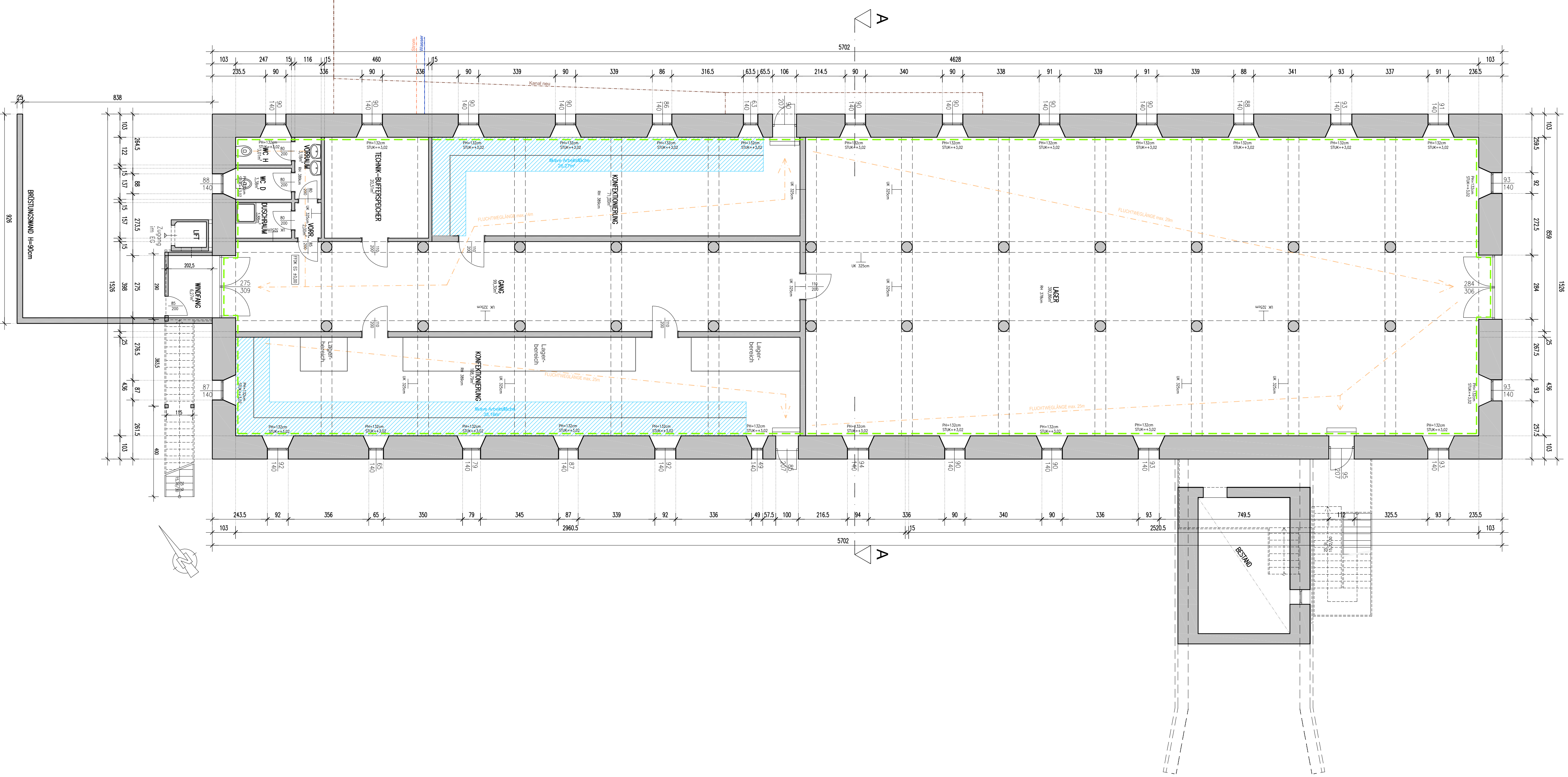
OBERGESCHOSS 1:100
