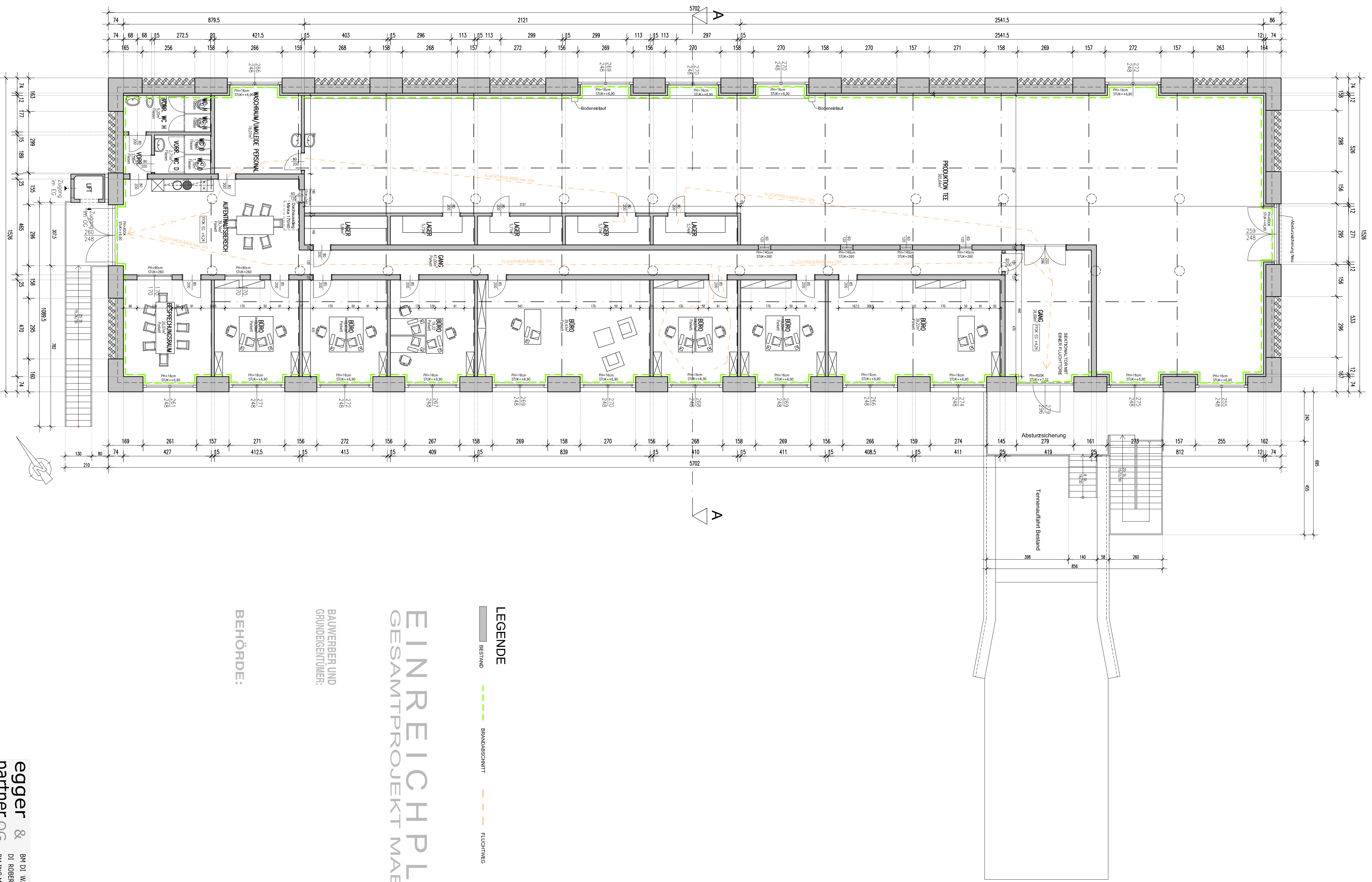
OBERGESCHOSS 1:100
