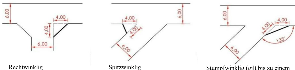
Abbildung 4 Abschrägung Parzellengrenzen in Kreuzungsbereichen
