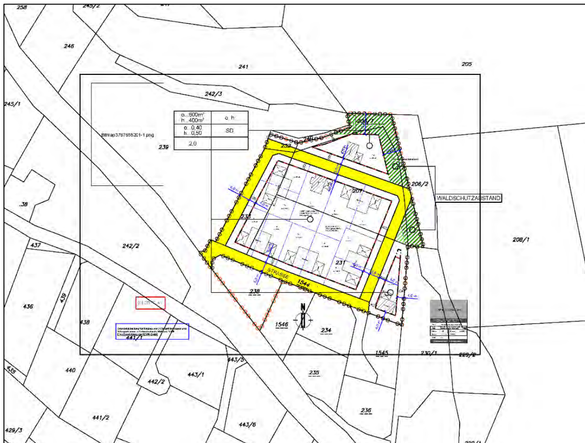
Abbildung 6: Aktuelles Bebauungskonzept (Quelle: Raumplanungsbüro LWK ZT-GmbH)
