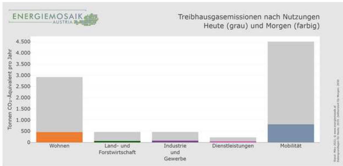
Abbildung 11: Treibhausgasemissionen bis 2050 7
