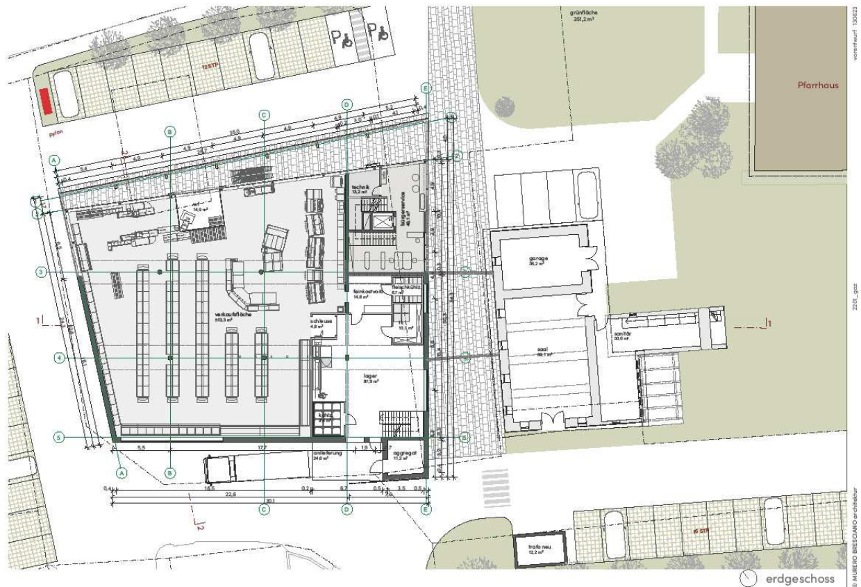
Abb. Erdgeschoss (Quelle: MURERO BRESCIANO architektur ZT GmbH)
