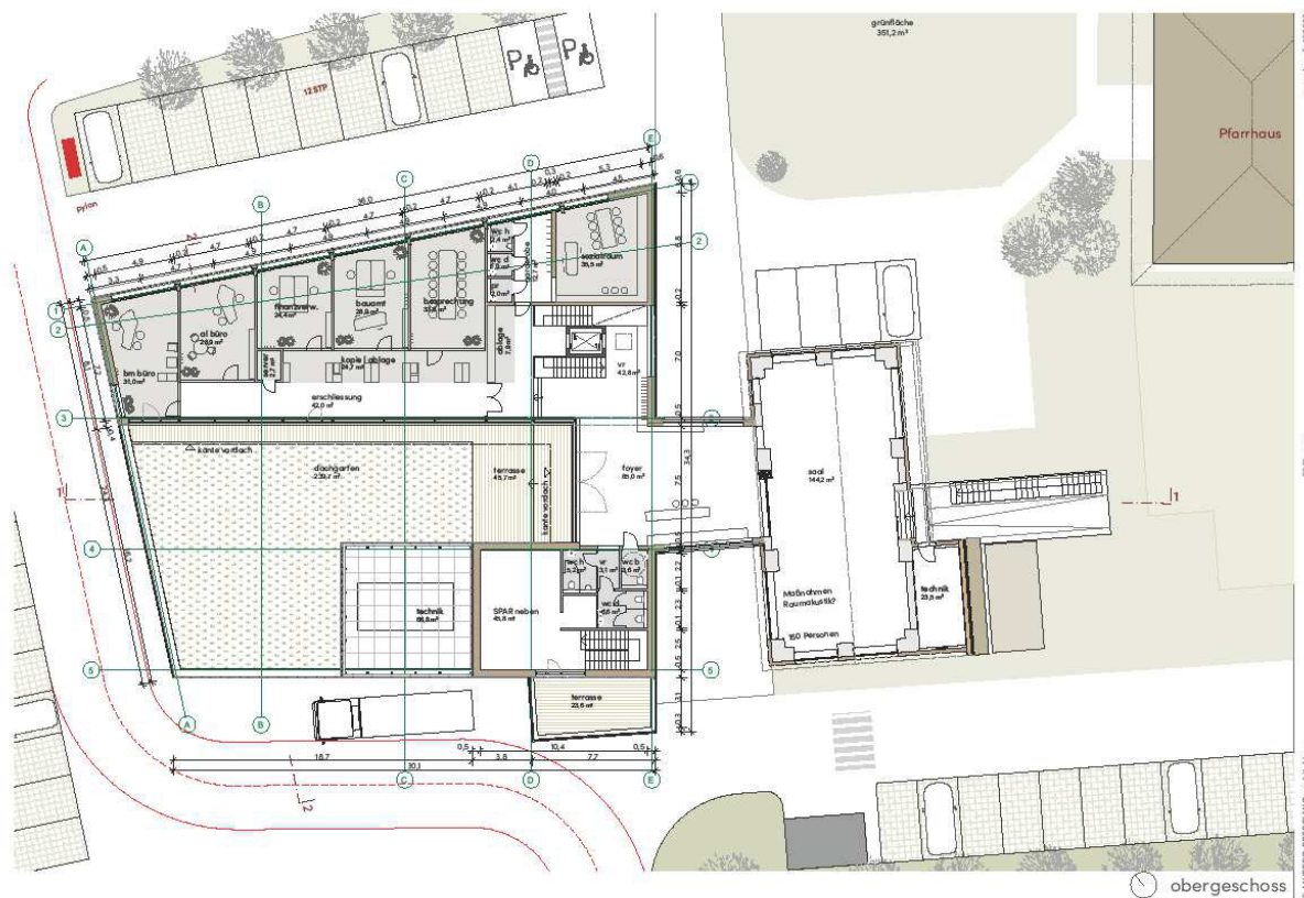
Abb. Obergeschoss (Quelle: MURERO BRESCIANO architektur ZT GmbH)
