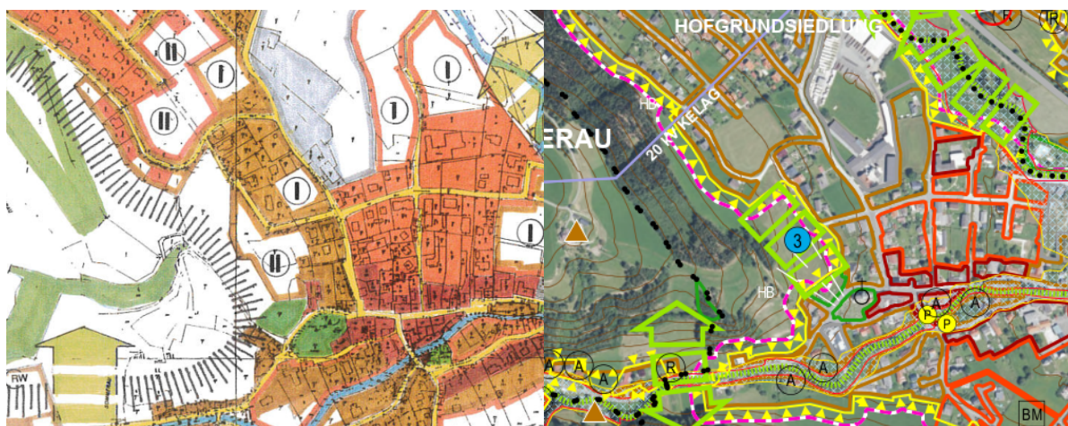
Abbildung 7-3: Gegenüberstellung Plansituation ALT (links) und NEU (rechts) – Bereich Pfarrkirche Reichenfels
